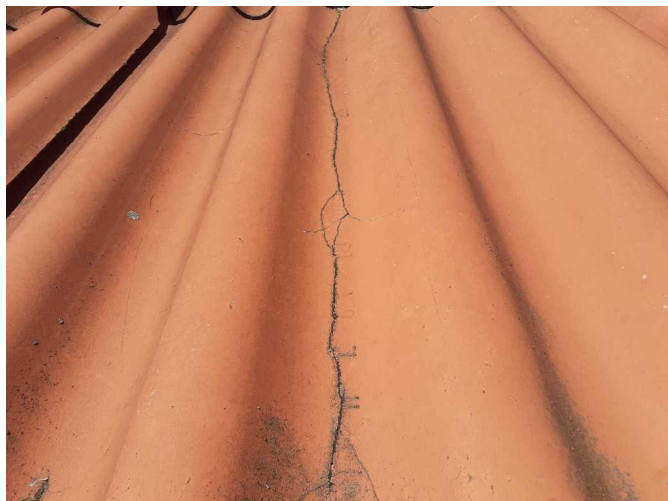
Foto /8/ Degradace střešní vlnité krytiny
