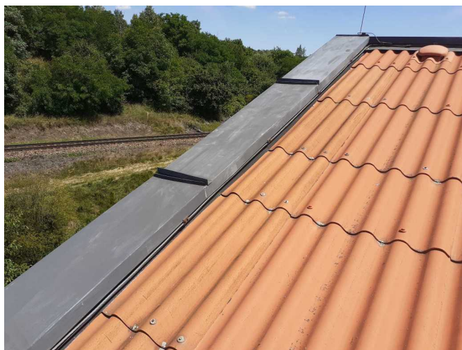
Foto /12/ Vnitřní okraj střechy v oblasti štítu
