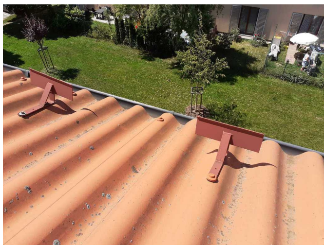
Foto /14/ Sněžové háky na okraji střechy
