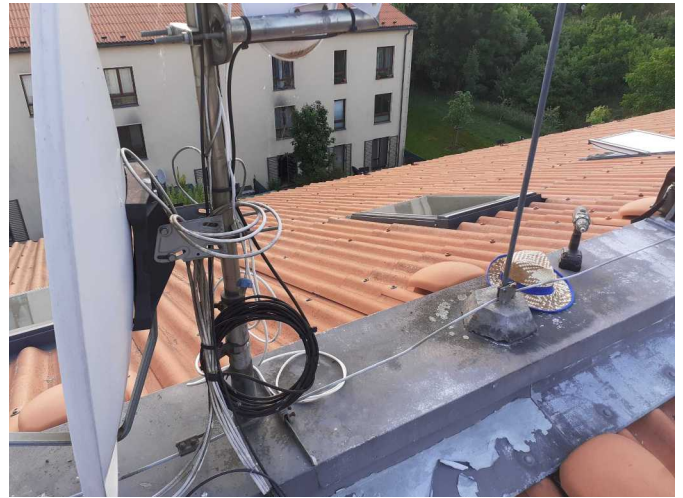
Foto /30/ Anténní stožár v hřebenové atice střechy
