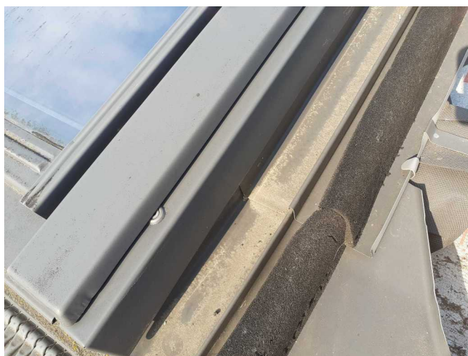
Foto /20/ Detail lemování střešního kyvného okna
